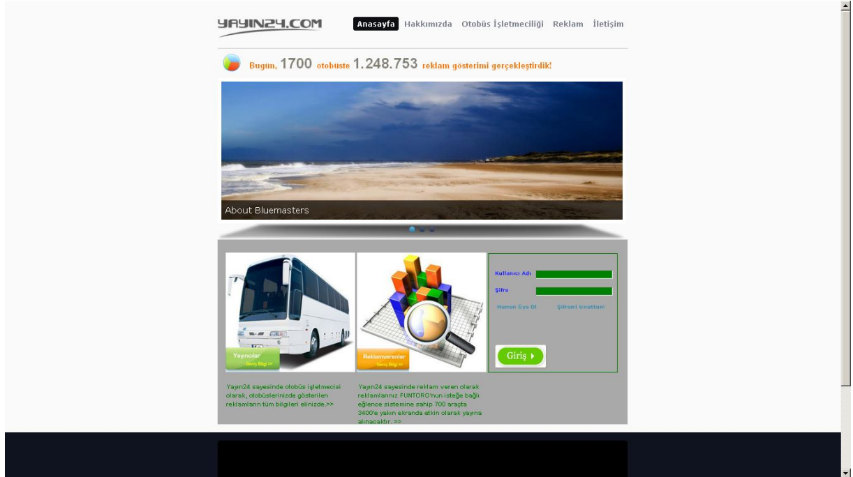
Şekil2-Giriş ekranı
