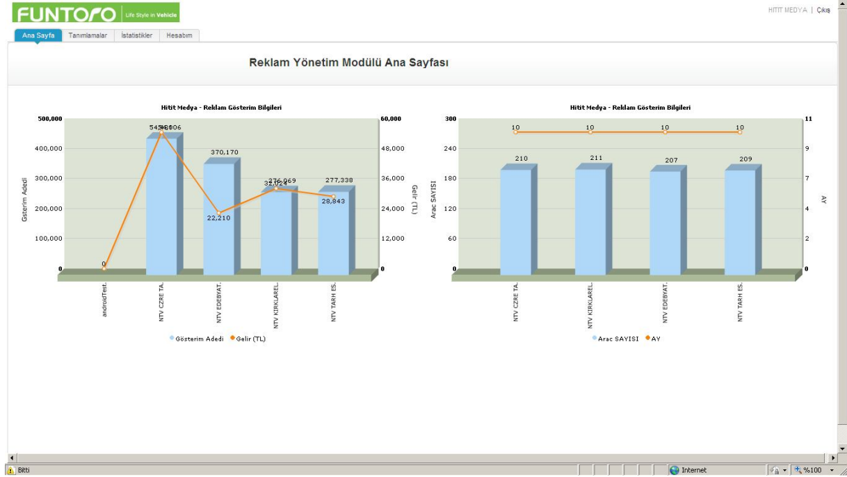
Şekil3-Ana Sayfa
